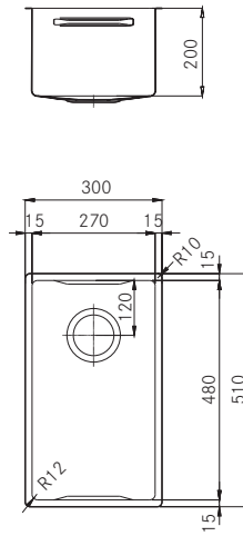
BWX 210/110 27
