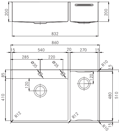
BWX 220 54-27 TL
